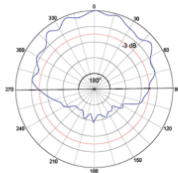
Horizontal Beamwidth
