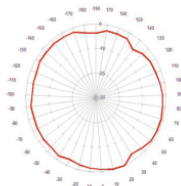
Horizontal Beamwidth
